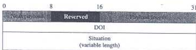
Figure 18.31 SA payload
