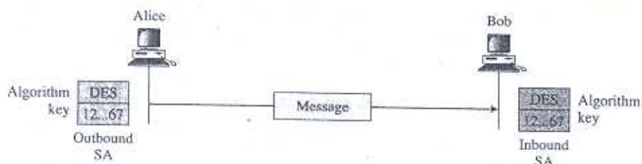
Figure 18.10 Simple SA
