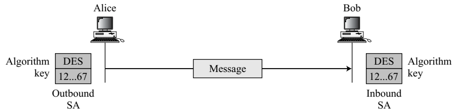
Figure 18.10 Simple SA
